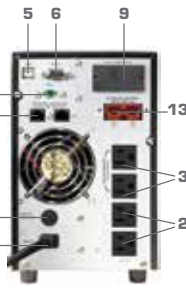
E4 LCD (S) Nema 1-1,5 kVA
