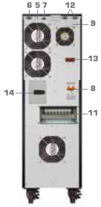
E4 LCD TX Nema 5-6-10(S) kVA
