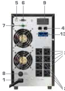
E4 LCD (S) Nema 2 kVA
